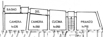
PIANO PRIMO
